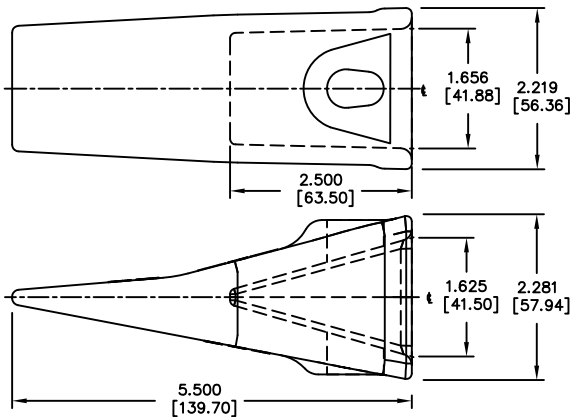
D6737325 2.3 lbs. (1.04 kgs.)
